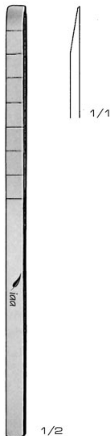
Cottle 02-755-18 4 mm 02-756-18 7 mm 02-757-18 9 mm 02-758-18 12 mm 18 cm / 7"
