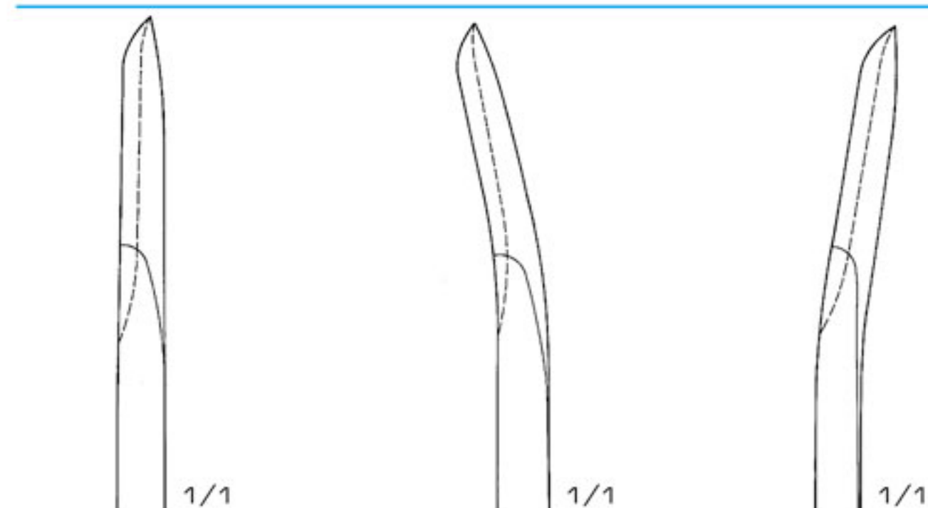
02-860-34 9 mm 02-863-34 9 mm 02-866-34 9 mm 02-861-34 15 mm 02-864-34 15 mm 02-867-34 15 mm 02-862-34 30 mm 02-865-34 30 mm 02-868-34 30 mm Inclined forward Inclined backward
