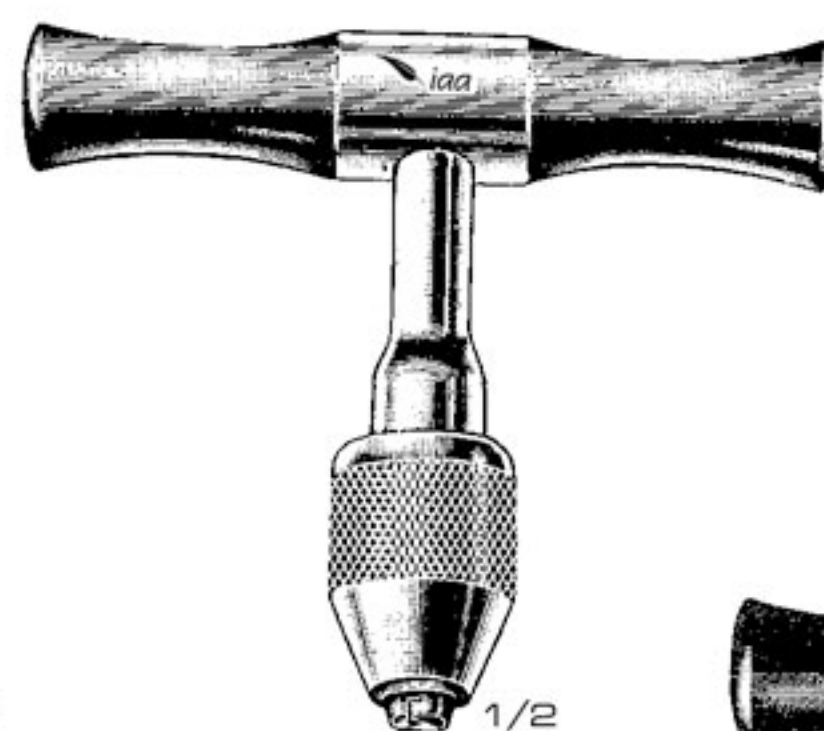
Stienmann 02-317-09 9 cm / 3¼"
