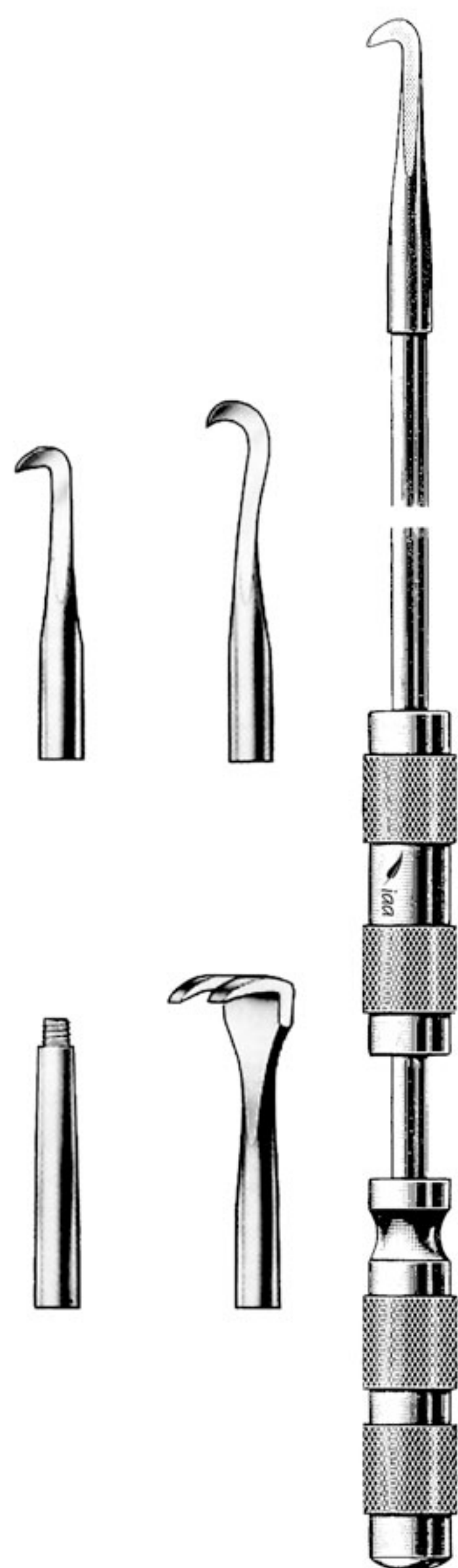
Kuntscher 02-402-45 45 cm / 17 3 / 4 " With 4 tips
