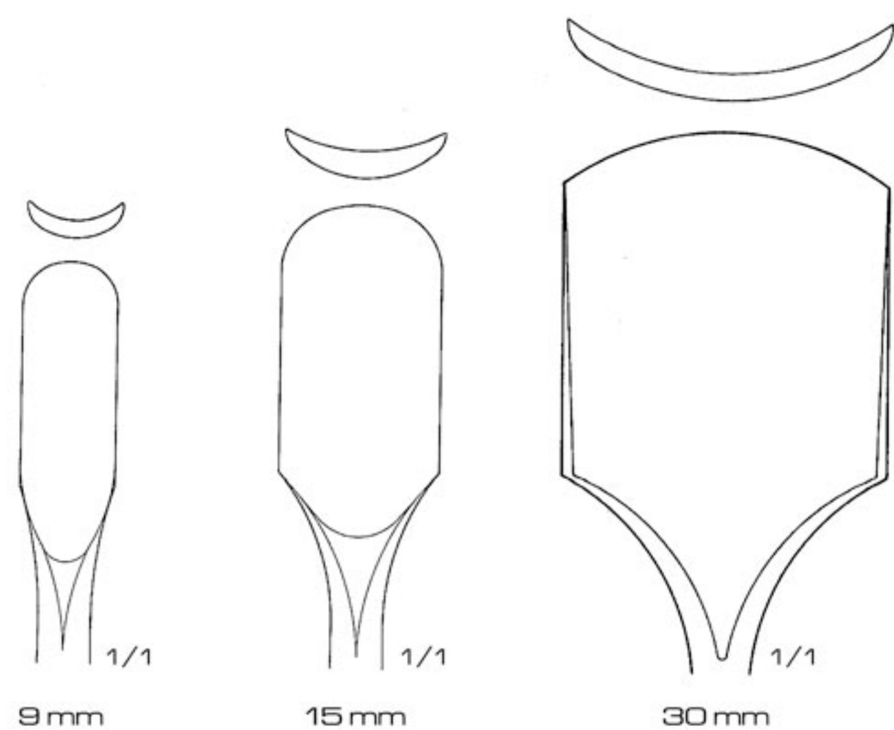
02-860-34 9 mm 02-863-34 9 mm 02-866-34 9 mm 02-861-34 15 mm 02-864-34 15 mm 02-867-34 15 mm 02-862-34 30 mm 02-865-34 30 mm 02-868-34 30 mm Inclined forward Inclined backward
